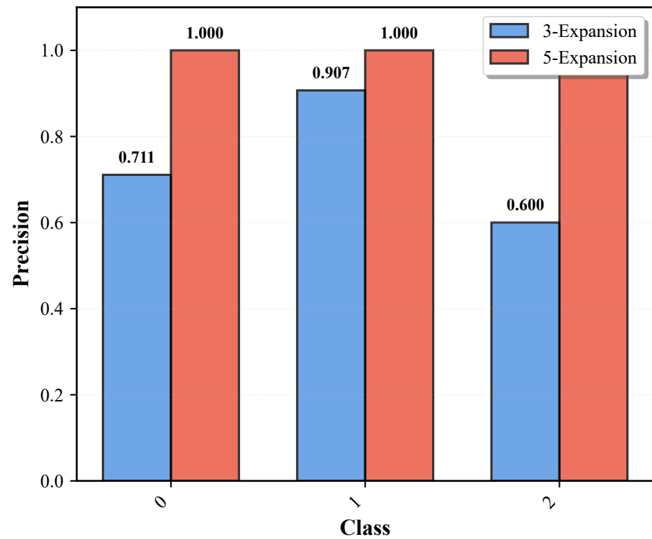
(a) Precision per Class
